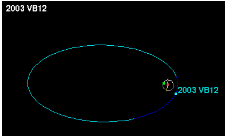
Fig. 7 – L'orbita di Sedna rispetto a quella (piccina) di Plutone.
