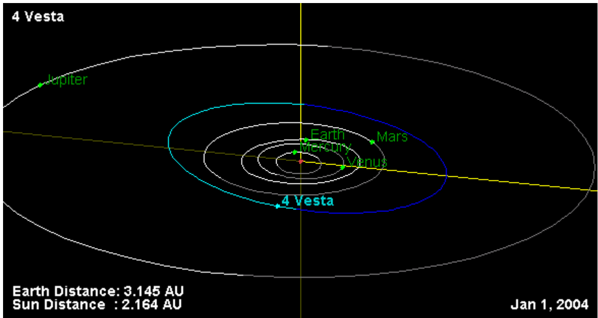
Fig. 5 – L'orbita di Vesta.
