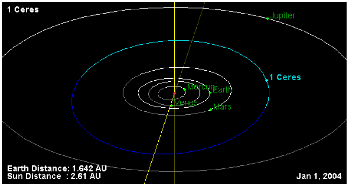
Fig. 3 – L'orbita di Cerere.
