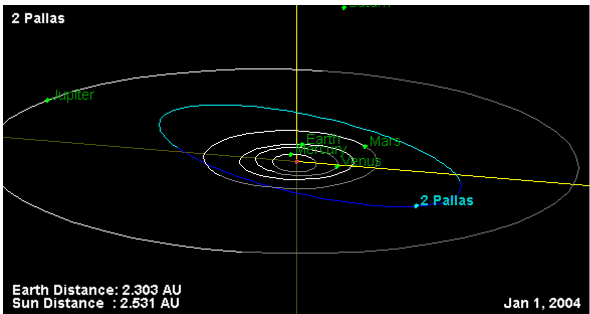
Fig. 4 – L'orbita di Pallade.
