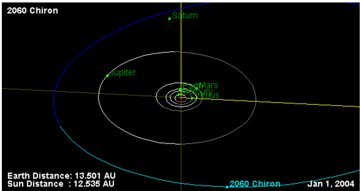
Fig. 6 – L'orbita di Chirone.
