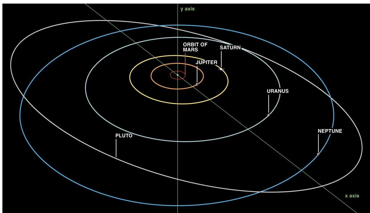
Fig. 2 – Il Sistema Solare oltre l'orbita di Marte.
